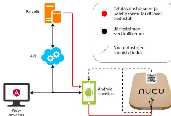
KUVA 2. Järjestelmän tietoliikenne
